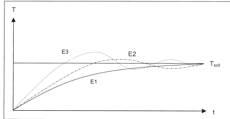
Abb.5: Regelverhalten der einzelnen Energie-Werte (schematisch) |
